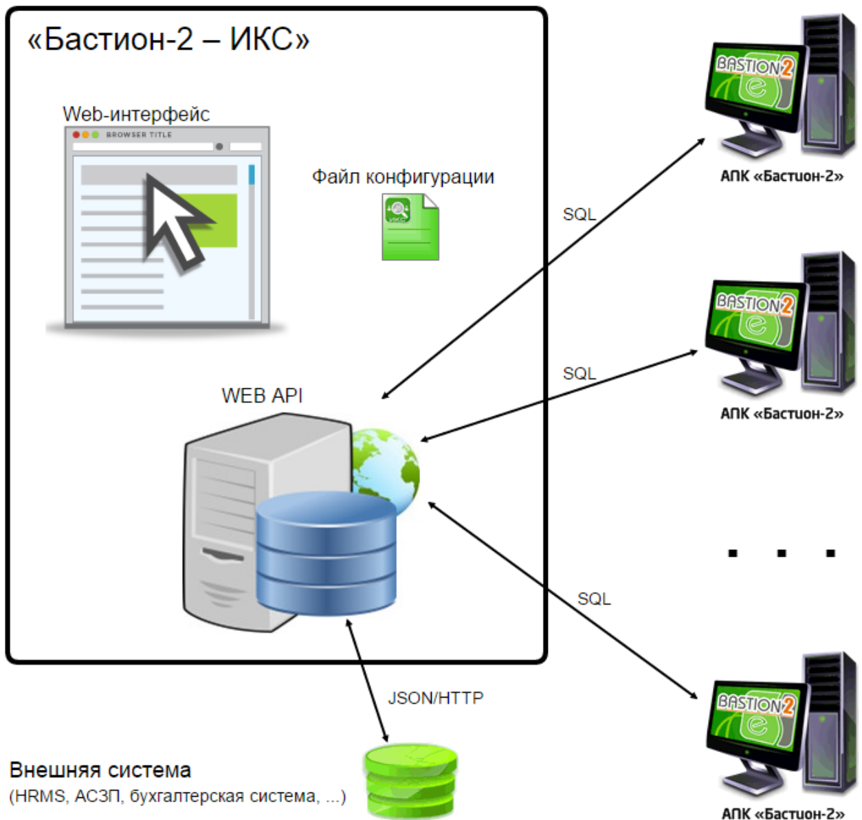
Рис. 1. Структура и схема взаимодействий модуля «Бастион-2 – ИКС»
