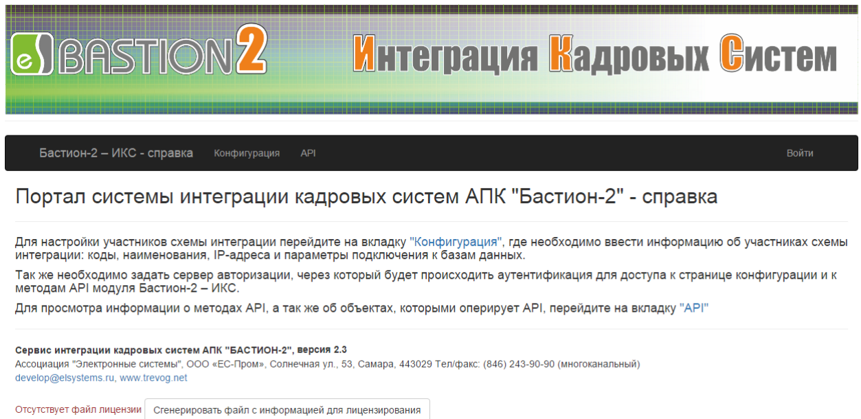
Рис. 5. Web-интерфейс
