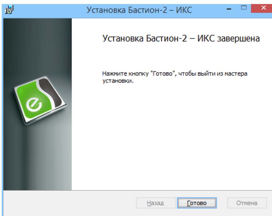
Рис. 3. Завершение установки
