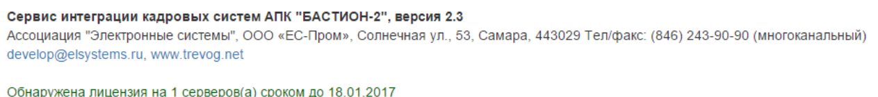
Рис. 7. Обнаружена лицензия
